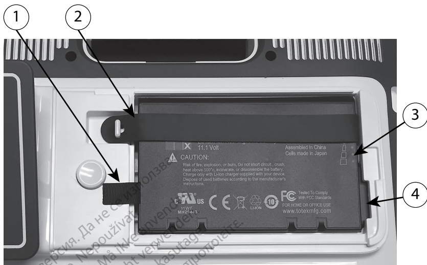
[1] Baterijas pacelšanas cilpa [2] Baterijas fiksēšanas sikсна [3] Baterijas stāvokļa indikatori [4] Baterijas savienotāja spāiles (daļēji paslēptas)
