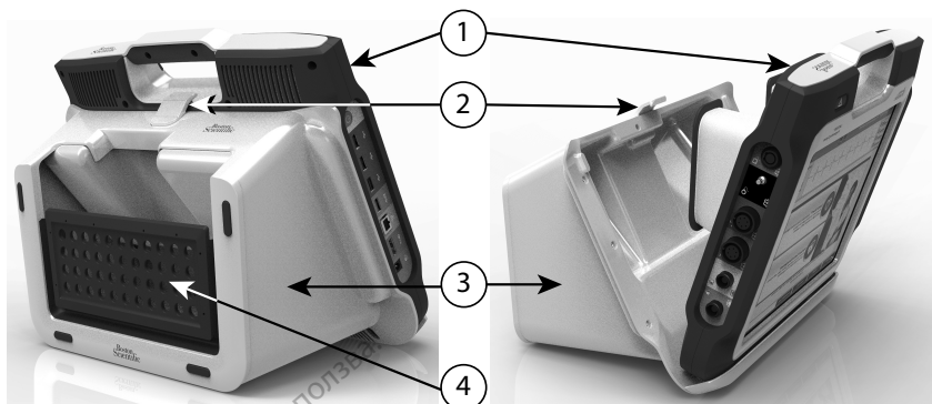
[1] 3300-as programozó [2] Tartó rögzítőkapcsa [3] 6755-ös tartó [4] Tárolószob
