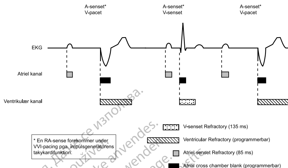
Figur 4-38. Refraktærperioder, VVI-pacemodus
