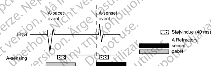
Figur 4-41. Refraktærperioder og støjvinduer, RA
