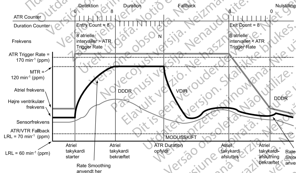
Figur 4-29. ATR-adfærd
