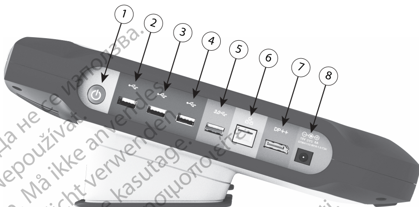
[1] Aan/uit-knop (lichtgrijs) [2-4] USB 2.0-poorten (donkergrijs) [5] USB 3.0-poort (blauw) [6] Ethernetpoort (oranje) [7] DisplayPort uit (rood-oranje) [8] Aansluiting gelijkspanning voor voedingsadapter model 6689 (groen)
