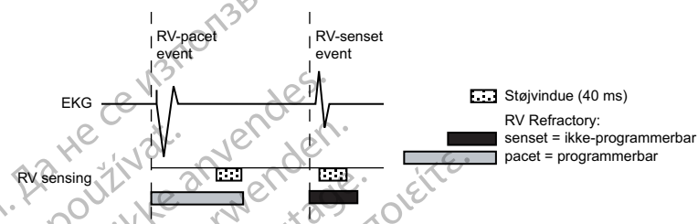
Figur 4-41. Refraktærperioder og støjvinduer, RV
