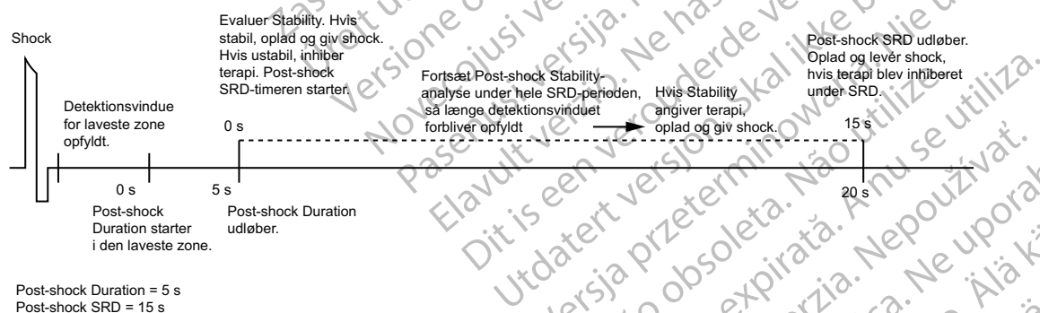
Figur 2–2. Analyse af Post-shock Duration og Post-shock Stability
