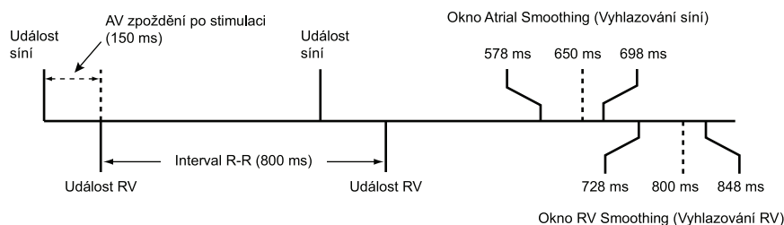
Obrázek 4-31. Okno synchronizace funkce Rate Smoothing (Vyhlažování frekvence)
