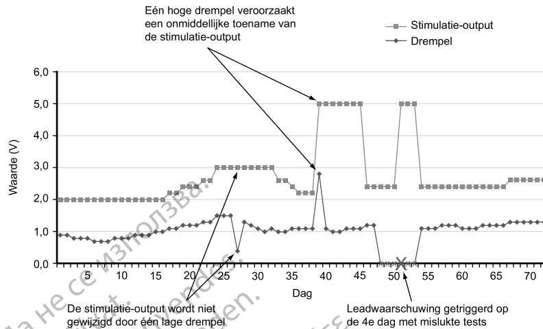
Figuur 4-6. Impact van drempelwijziging op RAAT-stimulatie-output
