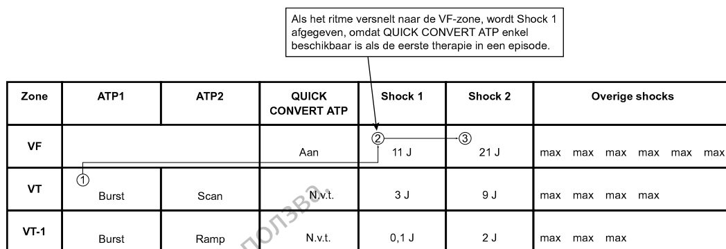
Figuur 3–10. Verloop van therapieafgifte, ATP1 in VT-zone verhoogt het ritme, QUICK CONVERT ATP wordt overgeslagen in VF-zone
