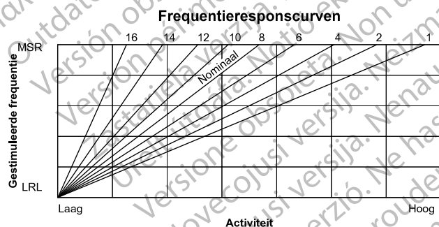
Figuur 4–9. Responsfactor en gestimuleerde frequentie
