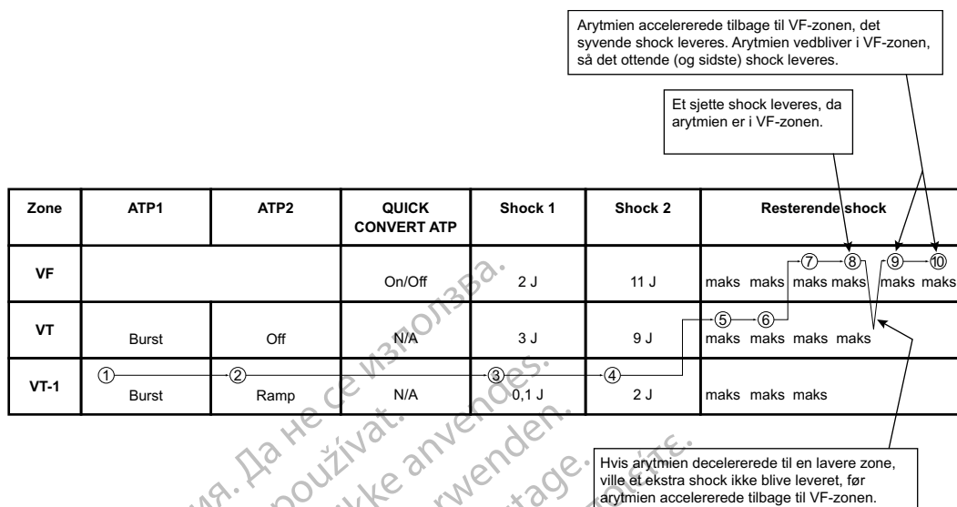
Figur 3-7. Forløb af terapilevering, sjette shock leveret
