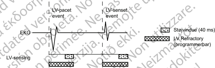
Figur 4-52. Refraktærperioder og støjvinduer, LV
