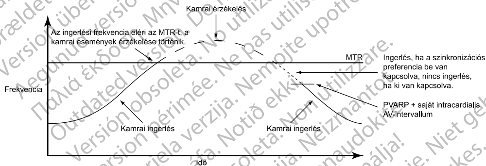
4-33. ábra Követési preferencia olyan pitvari események esetében, amelyeket követni kellene, de a PVARP-n belül esnek
