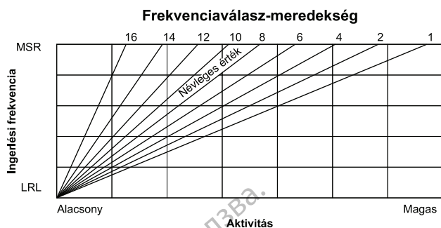
4-11. ábra A válaszfaktor és az ingerlési frekvencia
