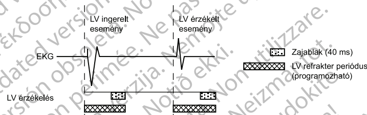
4-52. ábra Refrakter időszakok és zajablakok, LV
