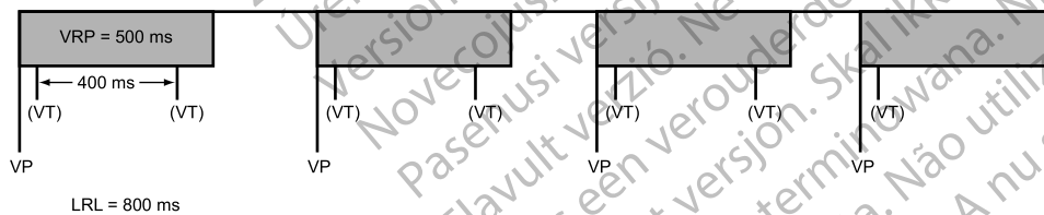
4–55. ábra Kamrai alulérzékelés VRP miatt
