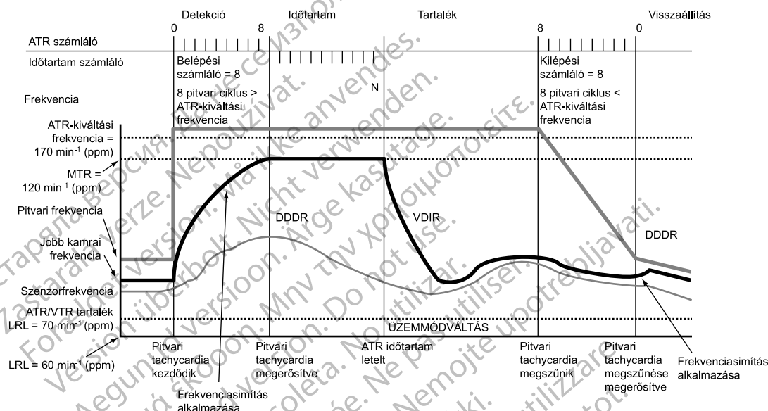
4–32. ábra Az ATR viselkedése
