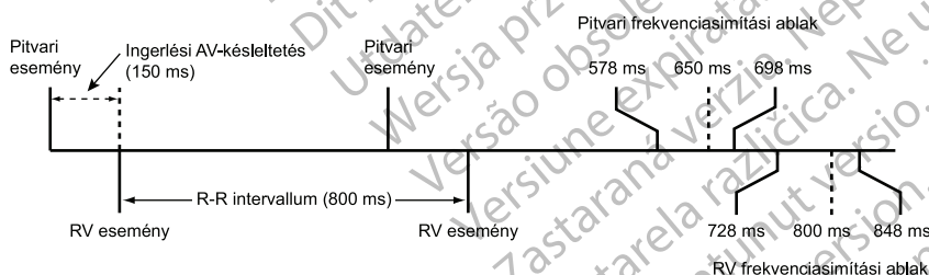
4–34. ábra Frekvenciasimítási szinkronizálási ablak
