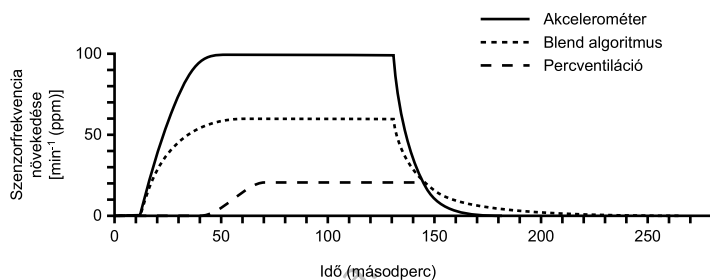
4-28. ábra Kombinációs válasz: Az akcelerométer mozgást érzékel, miközben az MV kis mértékben vagy nem emelkedik
