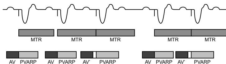
Figur 4-2. Wenckebach-adfærd ved MTR
