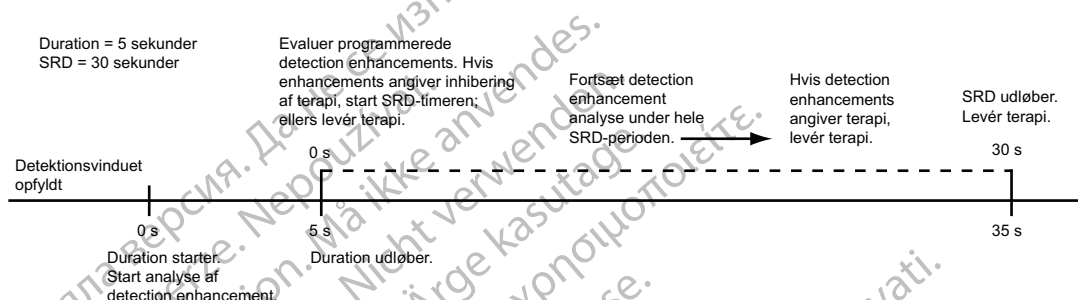
Figur 2-23. Kombination af Onset ELLER Stability, SRD programmeret til On
