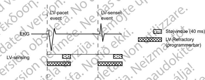
Figur 4-52. Refraktærperioder og støjvinduer, LV
