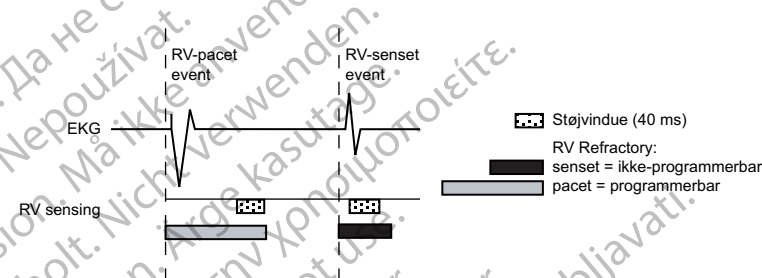
Figur 4-51. Refraktærperioder og støjvinduer, RV
