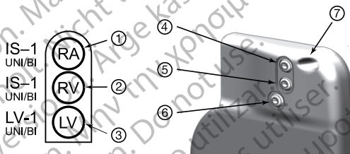
Figura 3. Collegamenti dell'elettrocatteter e posizione delle viti, AD: IS-1, VD: IS-1, VS: VS-1
