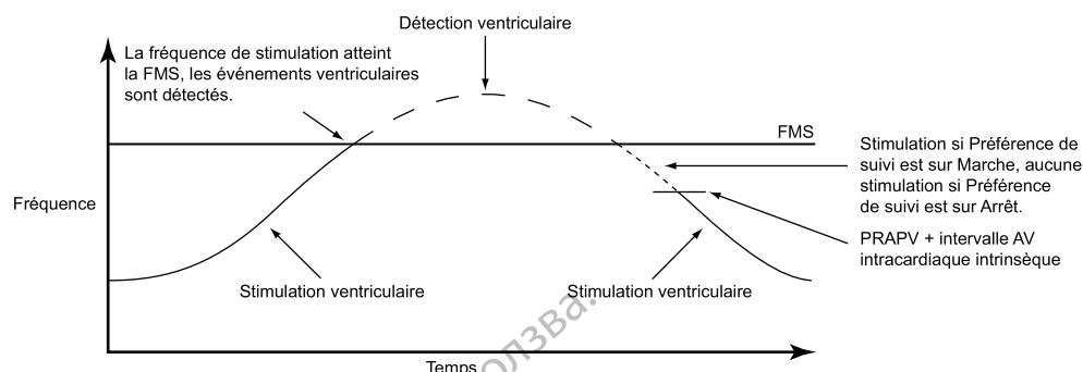
Figure 2-41. Préférences de suivi concernant les événements atriaux à suivre mais survenant durant la PRAPV
