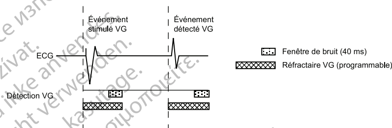
Figure 2-63. Périodes réfractaires et fenêtres de bruit, VG
