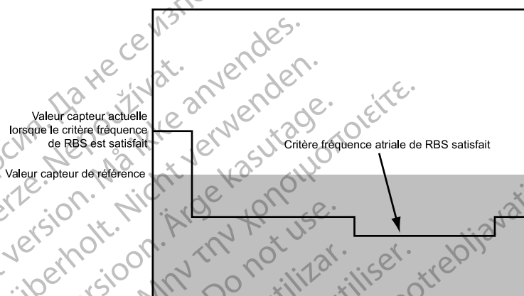
Figure 2–44. Traitement RBS inhibé durant la comparaison des capteurs
