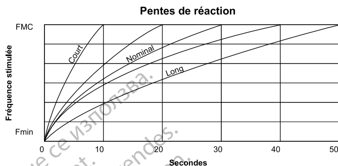
Figure 2-19. Temps de réaction et fréquence stimulée
