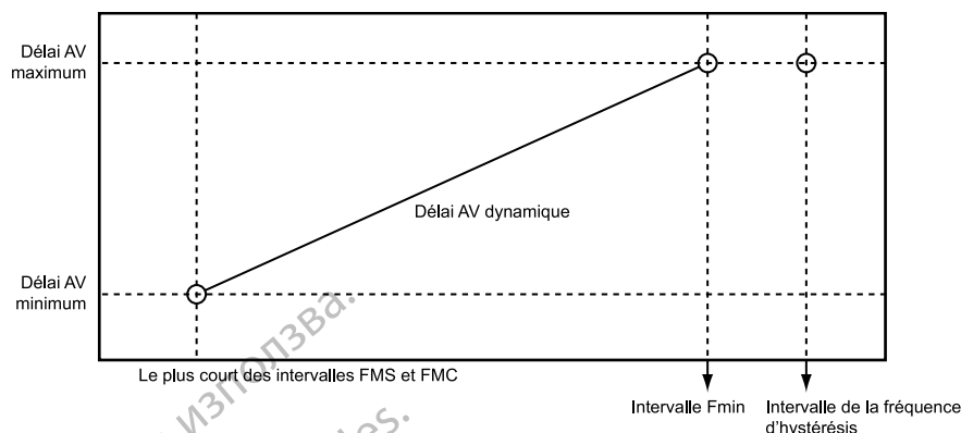
Figure 2-49. Délai AV dynamique
