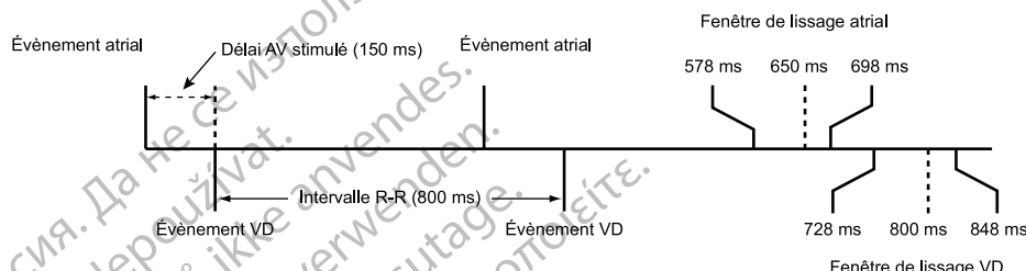
Figure 2-42. Fenêtre de synchronisation du lissage de fréquence
