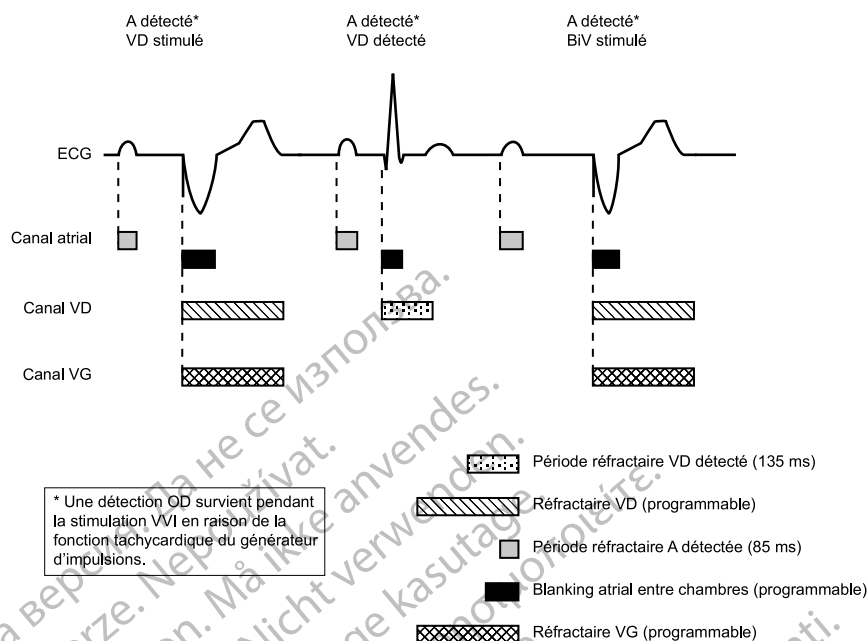
Figure 2-59. Périodes réfractaires, mode de stimulation VVI ; VD et BiV
