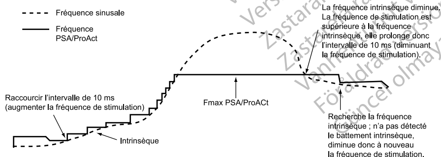
Figure 2-40. Préférence stimulation atriale
