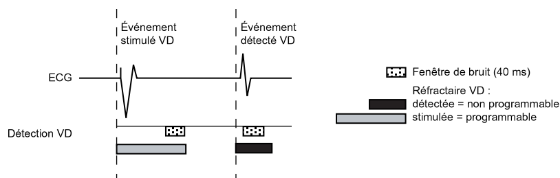
Figure 2-62. Périodes réfractaires et fenêtres de bruit, VD
