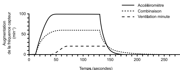
Figure 2-33. Réponse combinée : L'accéléromètre détecte un mouvement sans ou avec une très faible augmentation de la VM
