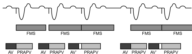
Figure 2-2. Comportement Wenckebach à la FMS
