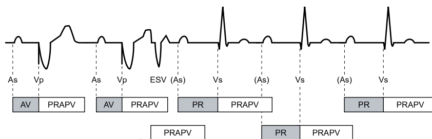
Figure 2-53. Événement atrial détecté en PRAPV
