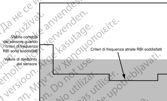
Figura 2-41. Terapia SBR inibita da Confronto con sensore
