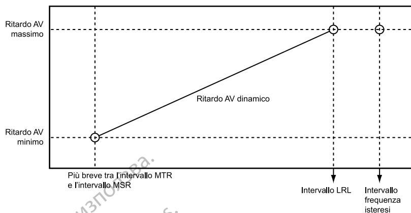
Figura 2-43. Ritardo AV dinamico
