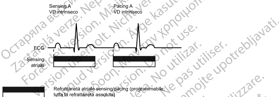
Figura 2-52. Periodi di refrattarietà, modalità di pacing AAI; SR
