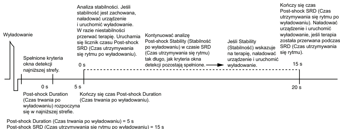
Ilustracja 2-2. Analiza parametrów Post-shock Duration (Czas trwania po wyladowaniu) i Post-shock Stability (Stabilność po wyladowaniu)
