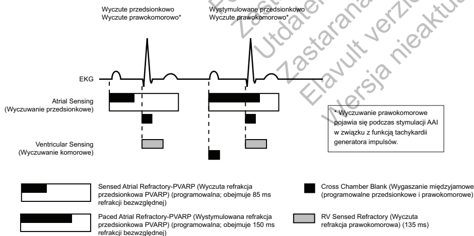
Ilustracja 4-39. Okresy refrakcji, tryb stymulacji AAI; DR
