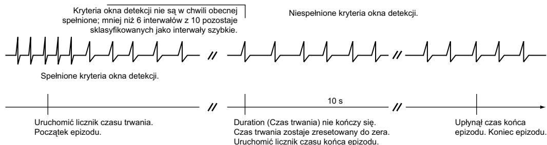
Ilustracja 2-14. Epizod nieleczoney, tryb komorowy Monitor + Therapy (Monitorowanie + terapia) lub Monitor Only (Tylko monitorowanie), nie upłynął czas trwania
