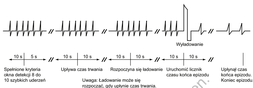
Ilustracja 6-2. Zależności między przechowywaniem EGM dla epizodu tachykardii komorowej a rejestrowaniem wykresu zapisu EKG powierzchniowego
