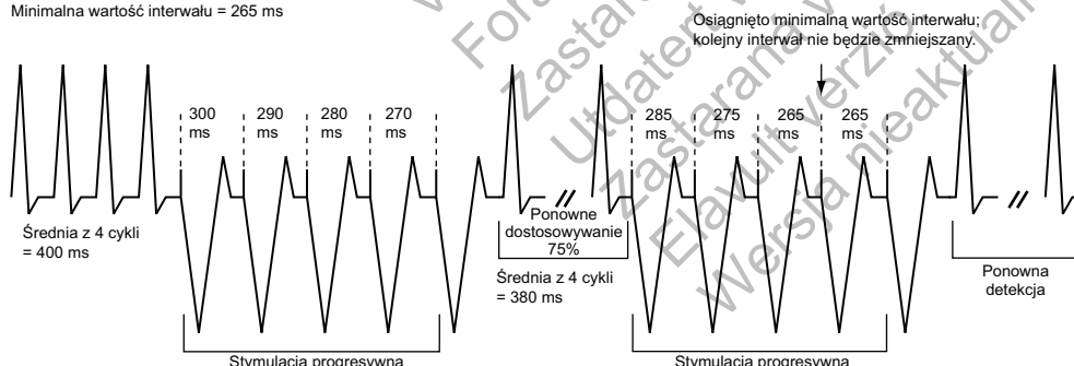
Ilustracja 3-16. Wartość 0 zaprogramowana dla parametrów Adaptive Ramp Scheme (Schemat stymulacji progresywnej z adaptacją), Coupling Interval Decrement (Zmniejszenie interwału sprzężenia) oraz Scan Decrement (Zmniejszenie skanowania)
