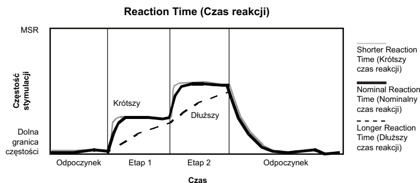
Ilustracja 4-14. Funkcja Reaction Time (Czas reakcji) w teście wysiłkowym
