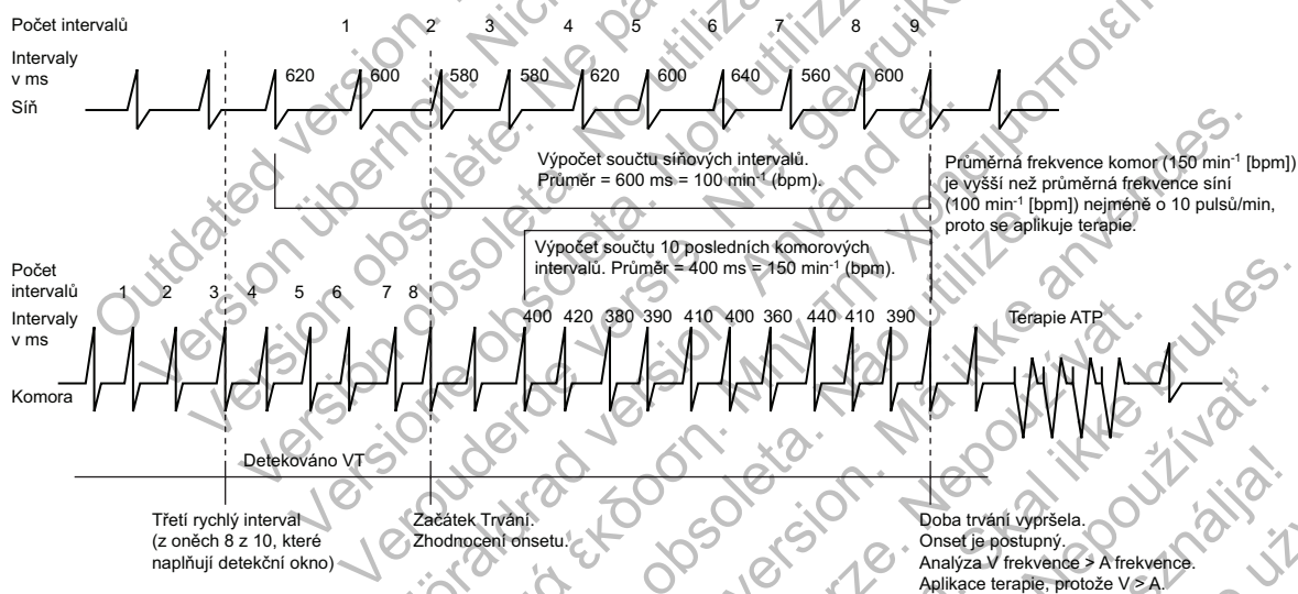
Obrázek 2-19. Analýza V \text{ Rate} > A \text{ Rate} (V frekvence > A frekvence)
