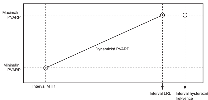
Obrázek 4-35. Možnost Dynamic PVARP (Dynamický PVARP)
