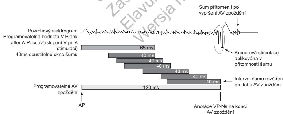
Obrázek 4-42. Noise Response (Odezva na šum) (pevně nastavené zaslepení)
