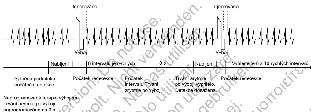
Obrázek 2-11. Redetekce po aplikaci komorového výboje
