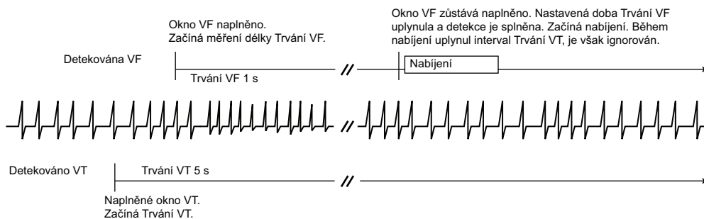
Obrázek 2-8. Interakce parametru Duration (Trvání) komor, 2-zónová konfigurace, nabíjení
