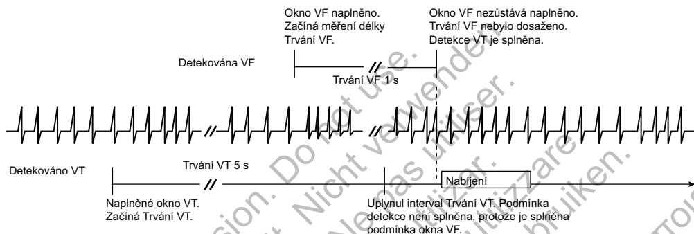
Obrázek 2-9. Interakce parametru Duration (Trvání) komor, 2-zónová konfigurace, zpožděné nabíjení
