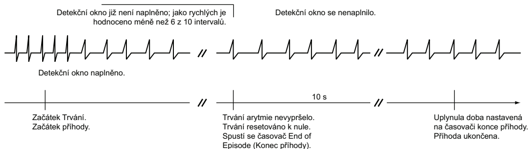
Obrázek 2-14. Neléčená epizoda, komorový režim je Monitor + Therapy (Sledování + terapie) nebo Monitor Only (Pouze sledování) a neuplynulo zpoždění
