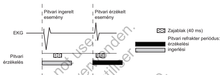
4-52. ábra Refrakter időszakok és zajablakok, RA
