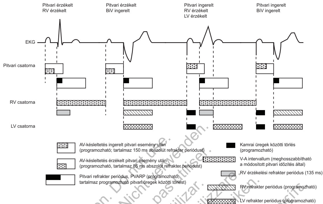
4-45. ábra Refrakter időszakok, kétüregű ingerlési módok; BiV
