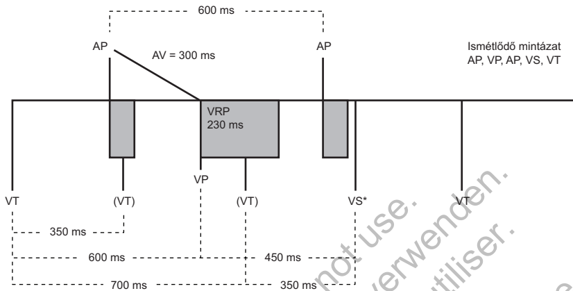
4-55. ábra Kamrai alulérzékelés pitvari ingerlés utáni kamrai törlés miatt
