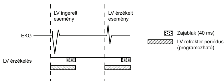
4-51. ábra Refrakter időszakok és zajablakok, LV
