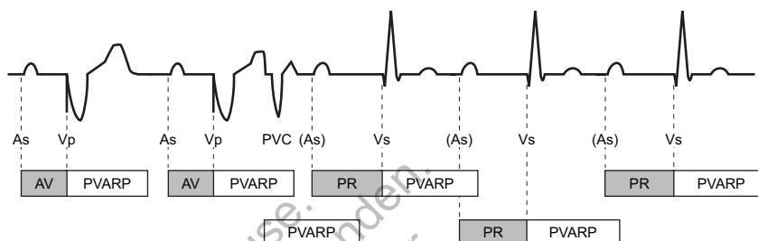
4-41. ábra Pitvari érzékelt esemény a PVARP időszakában
