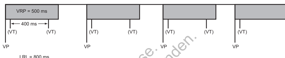
4-54. ábra Kamrai alulérzékelés VRP miatt
