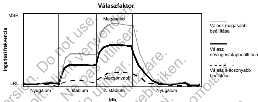
4-22. ábra A válaszfaktor beállításainak hatása egy kétfázisú terheléses próba során
