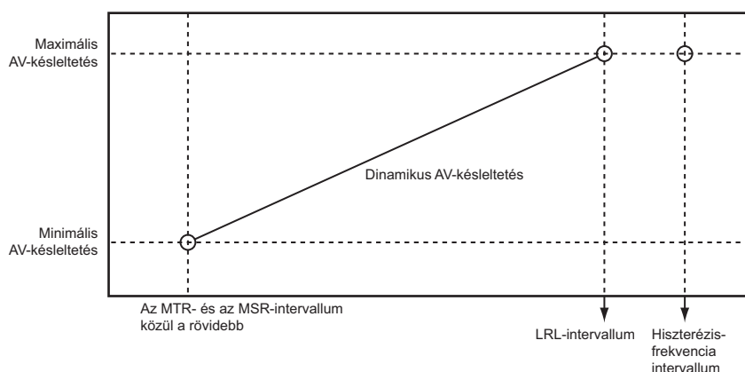
4-37. ábra Dinamikus AV-késleltetés
