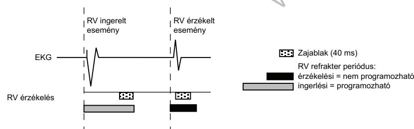
4-50. ábra Refrakter időszakok és zajablakok, RV
