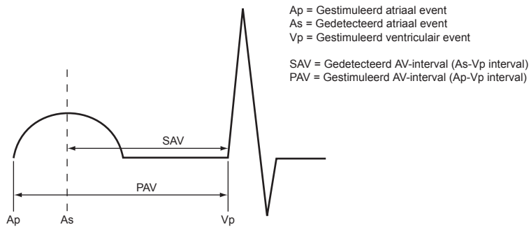
Figuur 4-38. Gedetecteerd AV-interval
