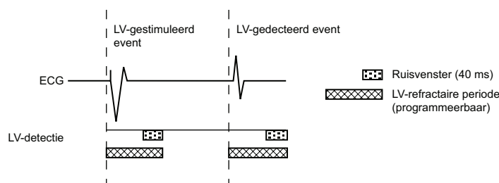
Figuur 4-51. Refractaire perioden en ruisvensters, LV
