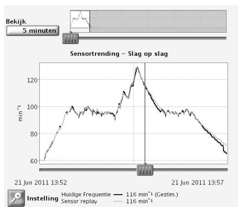
Figuur 4-30. Sensortrendinggrafiek
