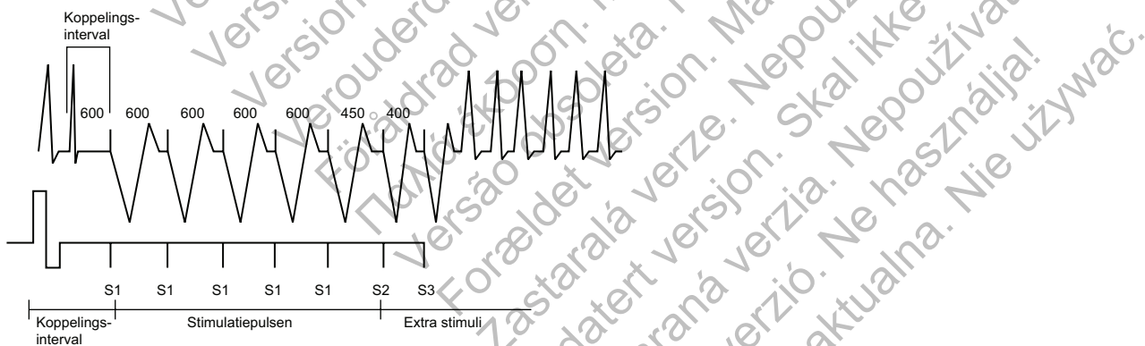
Figuur 7-3. PES-inductie pulstrein
