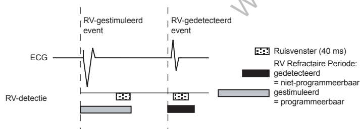
Figuur 4-50. Refractaire perioden en ruisvensters, RV
