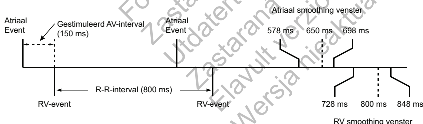
Figuur 4-33. Rate smoothing synchronisatievenster
