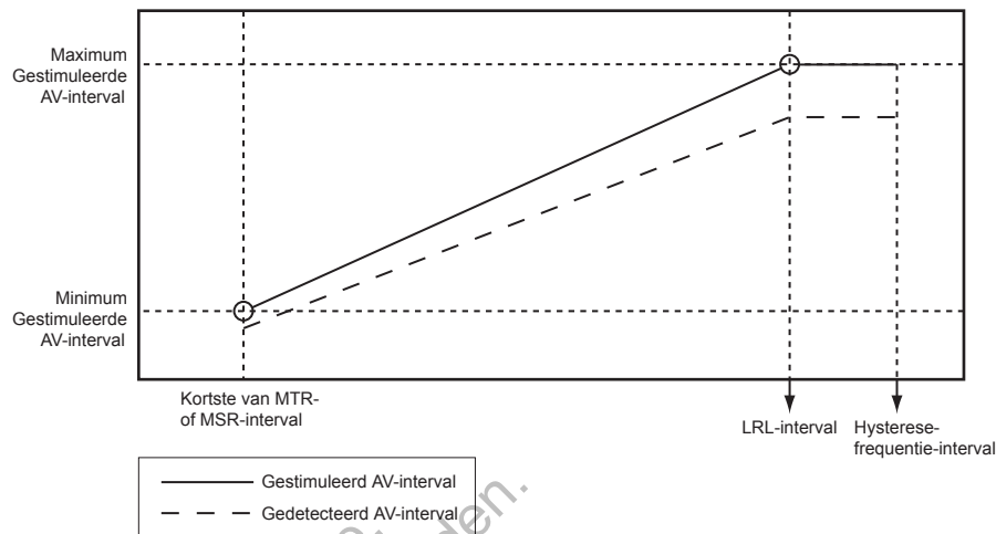
Figuur 4-39. Dynamische en Gedetecteerde AV-intervalfunctie
