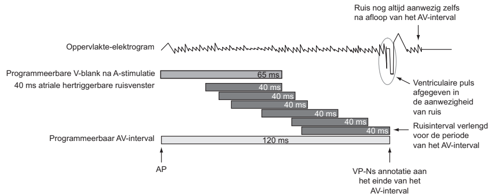
Figuur 4-53. Respons of ruis (vaste blanking)
