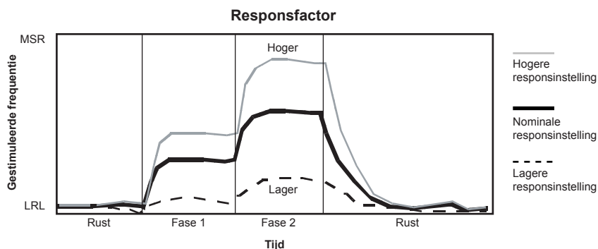
Figuur 4-12. Responsfactor tijdens inspanningstest
