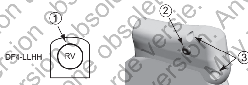
2. ábra A vezetékek csatlakozása és a rögzítőcsavarok elhelyezkedése, RA: IS-1, RV: DF4-LLHH
