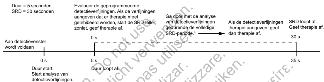
Figuur 2-23. Combinatie van Onset OF Stability, SRD staat aan
